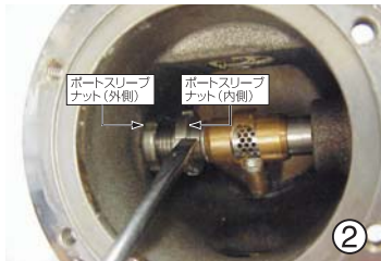
② マイナスドライバーでまずポートスリーブナット(外側)を反時計回りに、ポートスリーブナット(内側)を時計回りに廻して緩めて下さい。 ※ナットの切り込み部にマイナスドライバーをあてて軽くたたきながらはずして下さい。
